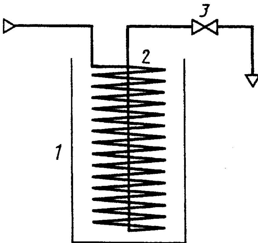
1 — сосуд для охлаждающей смеси; 2 — змеевик; 3 — игольчатый вентиль
